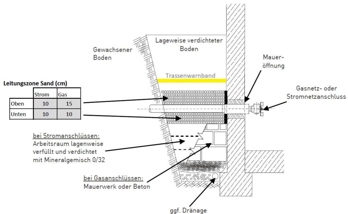
Abbildung: Unterbauung Netzanschluss im Bereich des Arbeitsraums
